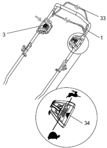
Управление скоростью автономного режима работы Рис. 9
